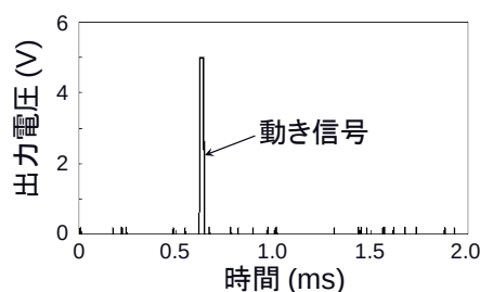
図 3 基本回路の時間応答
