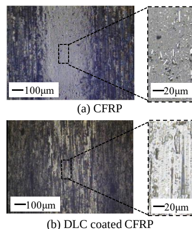
図2 CFRP と DLC コーティングを施した CFRP の摩耗痕の比較
