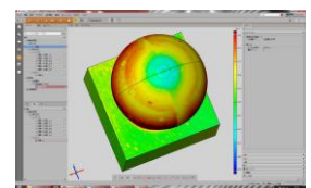
図3 3次元デジタイザによる精密測定
