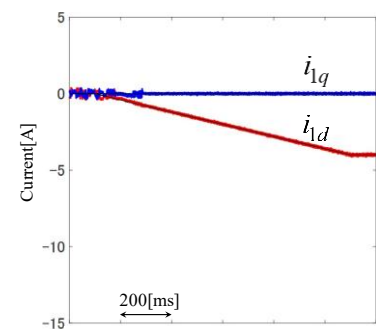
(b) 新規制御法の効果
